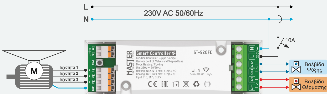
Διάγραμμα καλωδίωσης με Fan Coil 4 σωλήνων
